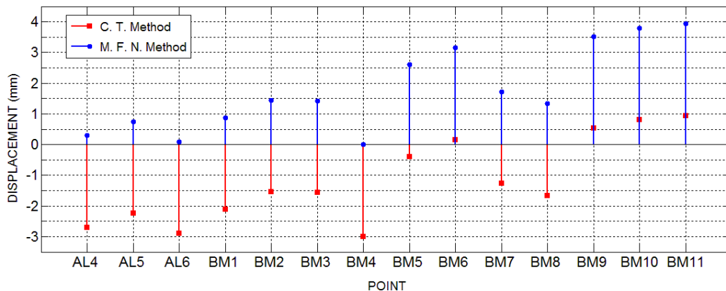
شکل ۳. جابه‌جایی نقاط مرجع بین ایگ‌های یکم و چهارم حاصل از روش‌های همانندی و مینیمم‌سازی نرم L_1 بردار جابه‌جایی
