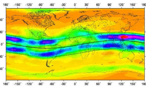
شکل ۵: مقدار توان طیفی پریود روزانه با ضریب 10^{-7} شکل ۶: مقدار توان طیفی پریود ۲۷ روزه با ضریب 10^{-3}
