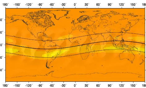
شکل ۷: مقدار توان طیفی پریود \frac{1}{4} سالانه با ضریب 10^{-4} شکل ۸: مقدار توان طیفی پریود \frac{1}{3} سالانه با ضریب 10^{-5}
