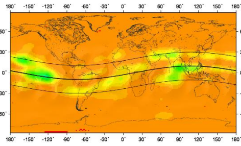
شکل ۱: مقدار توان طیفی پریود یک پنجم روزانه با ضریب 10^{-4} شکل ۲: مقدار توان طیفی پریود یک چهارم روزانه با ضریب 10^{-4}
