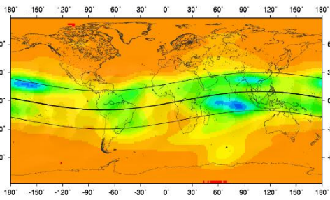
شکل ۳: مقدار توان طیفی پریود یک سوم روزانه با ضریب 10^{-5} شکل ۴: مقدار توان طیفی پریود یک دوم روزانه با ضریب 10^{-5}
