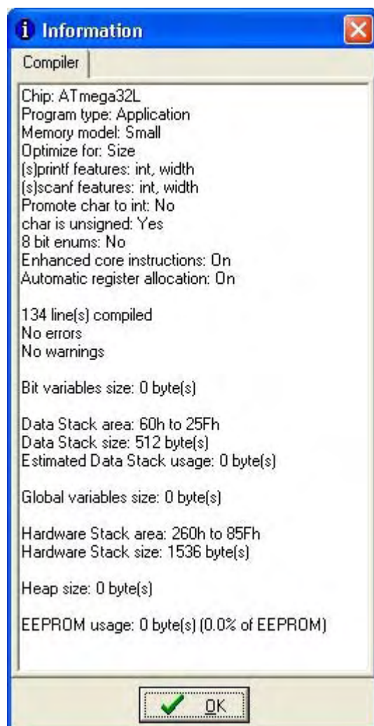
شکل ۳-۱۸ پنجره Information حاوی نتایج حاصل از کامپایل
